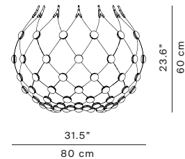
D86/D5
