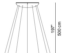
D86/D5
