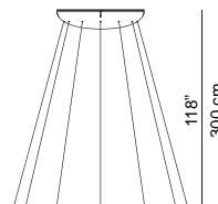
D86/D3
