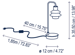
Through cord switch / Interruptor en el cable
